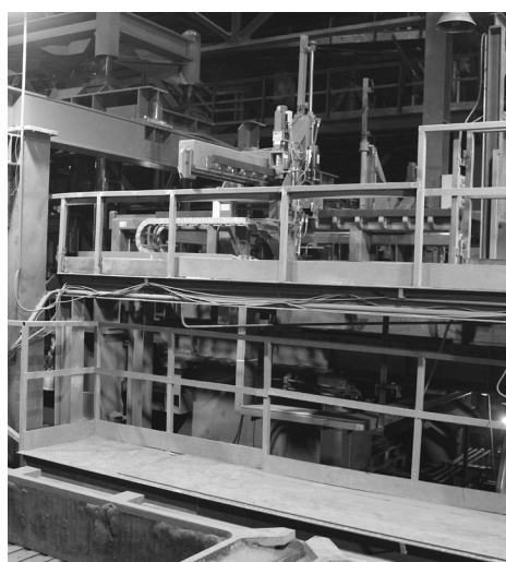
► Проведены монтажные работы устройства для прокалывания отверстий для выпоров в формах.
